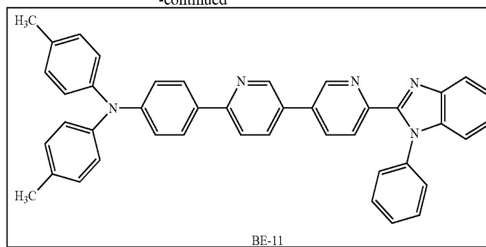
BE-11
