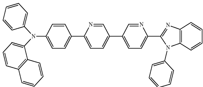
N-phenyl-N-(4-(6'-(1-phenyl-1H-benzo[d]imidazol-2-yl)-[3,3'-bipyridin]-6-yl)phenyl)naphthalen-1-amine, or
