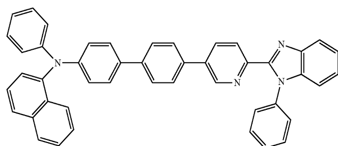
N-phenyl-N-(4'-(6-(1-phenyl-1H-benzo[d]imidazol-2-yl)pyridin-3-yl)-[1,1'-biphenyl]-4-yl)naphthanen-1-amine,
